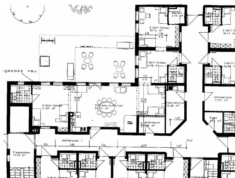
Abb. 31: Grundriss Pflegeoase
